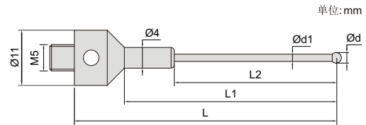
M5带台阶测针(不锈钢基座)
