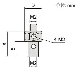
M2多路测针中心座 (mm)
