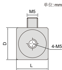
M5四路测针中心座
